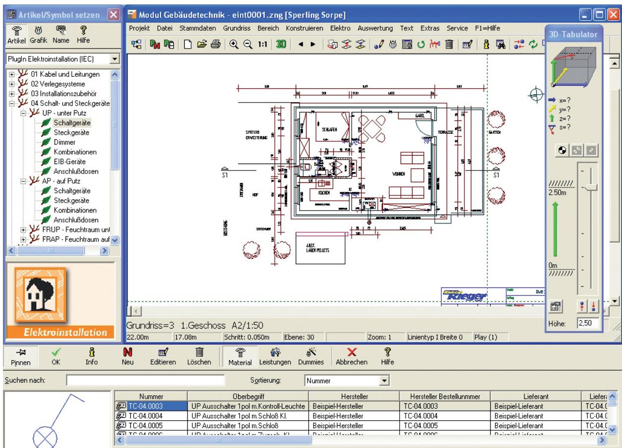
Abbildung: Beispielprojekt der Elektro Rieger GmbH, Projektiert mit Treesoft CAD Gebäudetechnik
